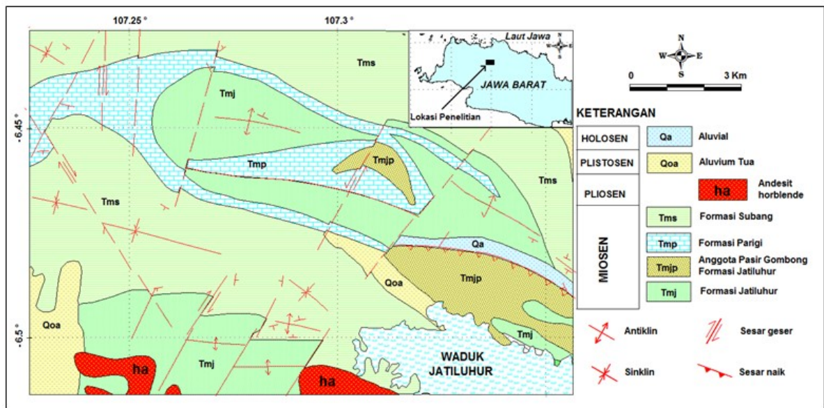
Gambar 1. Peta geologi daerah Karawang (Achdan dan Sudana, 1992)
